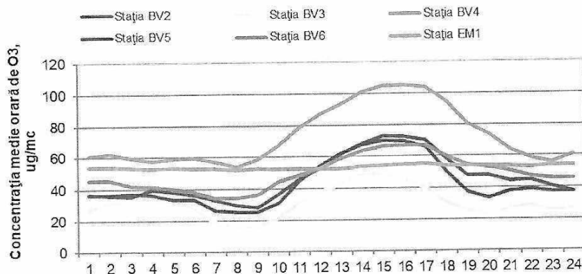
Figura 1.1.2.3.2. Ciclul zilnic al ozonului
