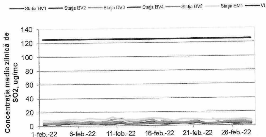
Figura 1.1.2.1.1. Evoluția mediilor zilnice de \text{SO}_2 în luna februarie
