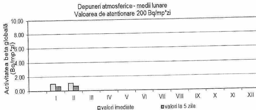
Fig. 1.2.4. Activitatea beta globală pentru depuneri atmosferice
